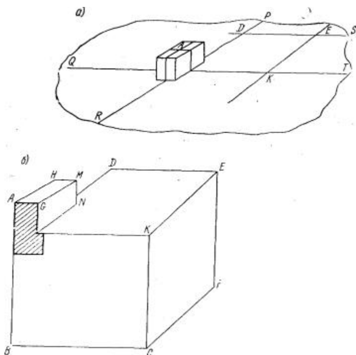
Рис. 34. Прямоугольный бетонный массив а - общий вид; б - расчетная область сооружения
