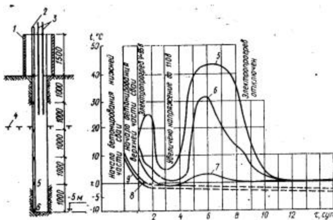
Рис. 54. Температурный режим остывания бетона в свае-модели диаметром 550 мм с электропрогревом
