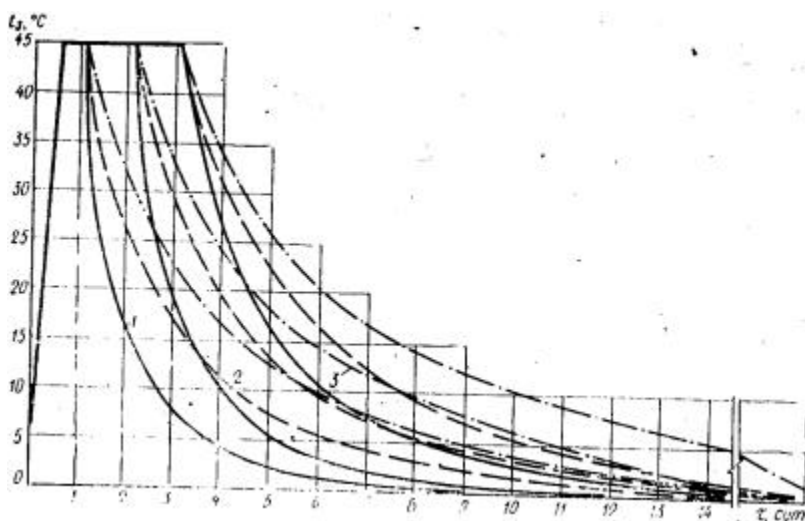
Рис. 16. Характер остывания конструкций, расположенных ниже деятельного слоя 1 - сваи диаметром 600 мм; 2 - то же, 1000 мм; 3 - то же, 1400 мм
