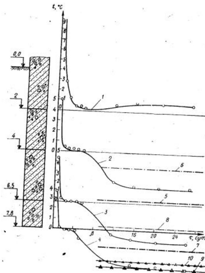
Рис. 53. Изменение температур во времени у поверхности железобетонной сваи 1 - на глубине 2 м; 2 - то же, 4 м; 3 - то же, 6,5 м; 4 - то же, 7,8 м; 5 - начальное распределение температур в грунте на глубине 4 м; 6 - естественное распределение температур в грунте на глубине 4 м в октябре (максимальные температуры); 7 - начальное распределение температур в грунте на глубине 6,5 м; 8 - естественное распределение температур в грунте на глубине 6,5 м в октябре (максимальные температуры); 9 - начальное распределение температур в грунте на глубине 7,8 м; 10 - естественное распределение температур в грунте на глубине 7,8 м в октябре (максимальные температуры)
