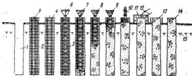
Рис. 8. Технологическая схема бетонирования буронабивных свай методом ВПТ
