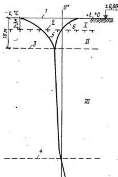
Рис. 1. Схема расположения зон грунта
