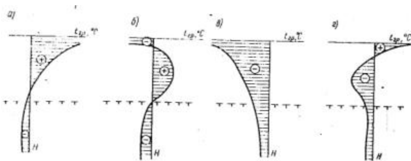
Рис. 14. Характер распределения температуры вечномерзлого грунта t_{гр} по глубине H в течение года
