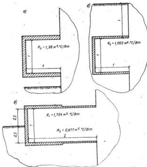
Рис. 41. Схемы бетонируемых выступов
