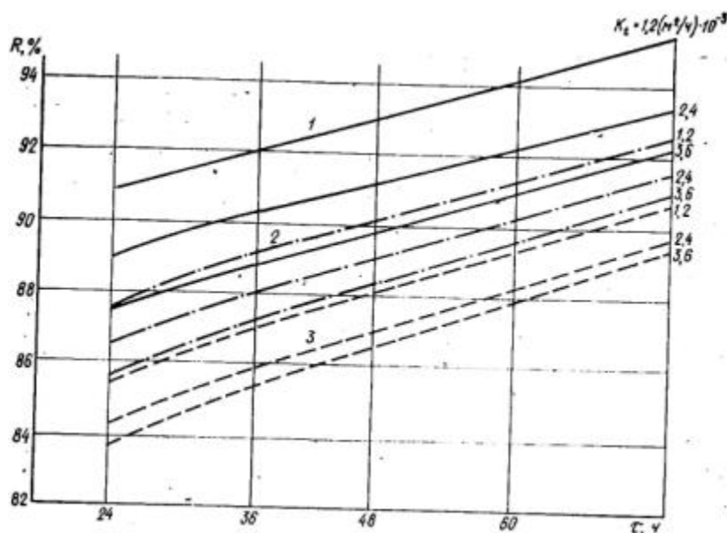
Рис. 15. Номограмма для определения прочности бетона, прогретого по различным режимам и выдерживаемого в грунтах с температурой от -1 до -5°C 1 - сваи диаметром 1400 мм; 2 - то же, 1000 мм; 3 - то же 800 мм
