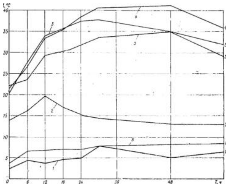
Рис. 10. График остывания бетона в обделке тоннеля 1 - температура воздуха; 2 - то же, на контакте бетон - опалубка; 3 - то же, на расстоянии 25 см от поверхности опалубки; 4 - то же, на расстоянии 50 см; 5 - то же, на расстоянии 75 см; 6 - то же, на расстоянии 1 м или на контакте бетон - порода
