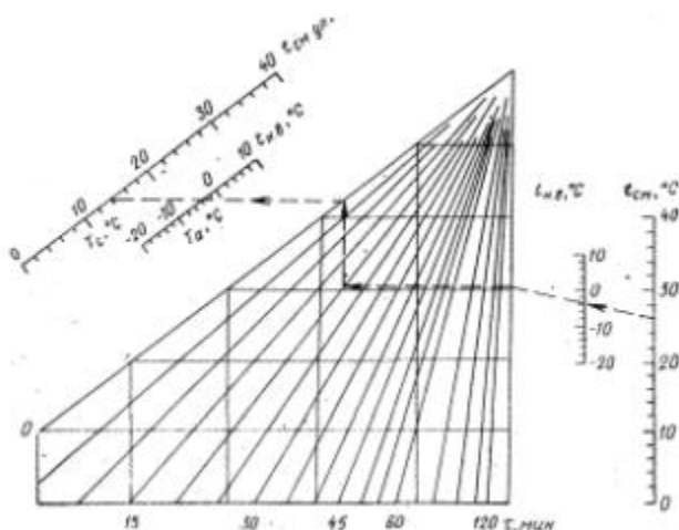
Рис. 4. Номограмма для назначения температуры бетонной смеси
