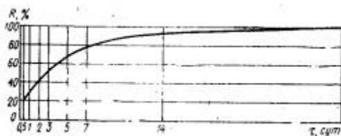
Рис. 44. График нарастания прочности, % R_{28} , бетона марок М 200 - М 300 на портландцементе марки М 400 при температуре 20°C
