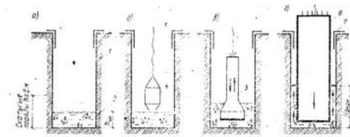
Рис. 13. Последовательность операций при омоноличивании пяты столбов фундаментов
