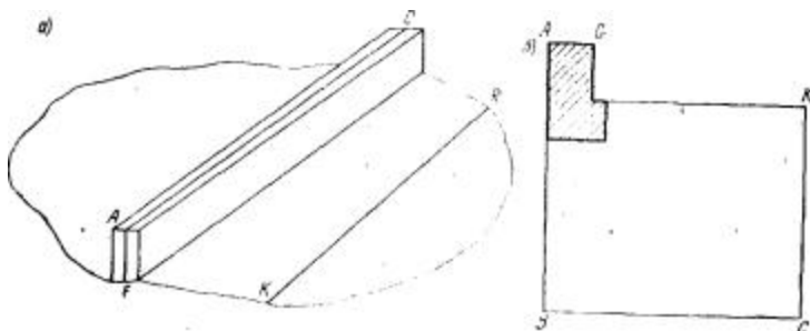
Рис. 35. Бетонная стенка а - общий вид; б - расчетная область сооружения
