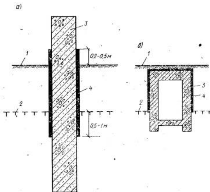
Рис. 3. Схема изоляции бетона в вечномёрзлых грунтах а - свал; б - коммуникационный канал; 1 - уровень грунта; 2 - верхняя граница вечномёрзлого грунта; 3 - бетон; 4 - гидроизоляция
