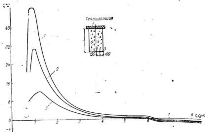
Рис. 55. Температурный режим остывания бетона, выдерживаемого комбинированным способом
