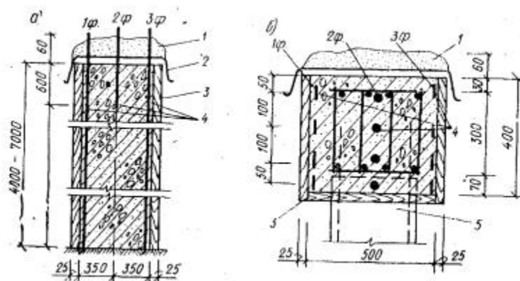
Рис. 49. Схема электропрогрева конструкций
