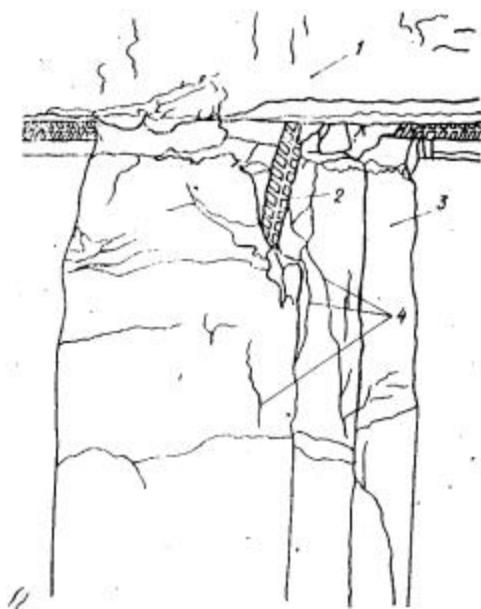
Рис. 18. Влияние температурно-влажностных деформаций на оголовки свай при низких отрицательных температурах 1 - ростверк; 2 - скол бетона и оголенная арматура сваи; 3 - свая; 4 - трещины в бетоне
