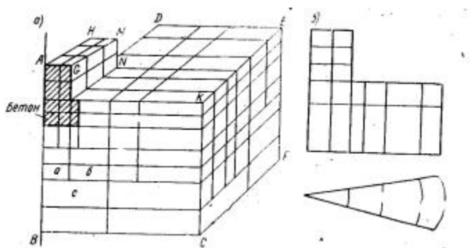
Рис. 37. Система разбивки на блоки расчетной области
