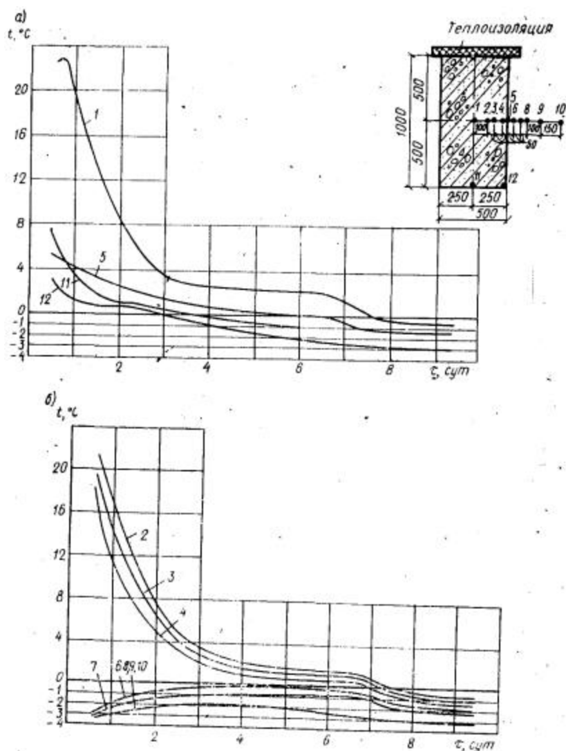
Рис. 50. Схема расположения термодар и температурный режим бетона в свае-модели диаметром 500 мм и прилегающего вечномёрзлого грунта а - в центре и углах бетона (номера термодар и кривых 1, 5, 11, 12); б - в бетоне и прилегающем грунте (соответственно номера термодар и кривых 2-4 и 6-10)
