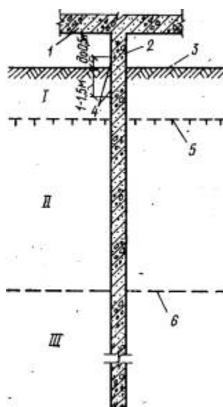
Рис. 2. Схема расположения элемента свайного фундамента в различных зонах вечномёрзлого грунта
