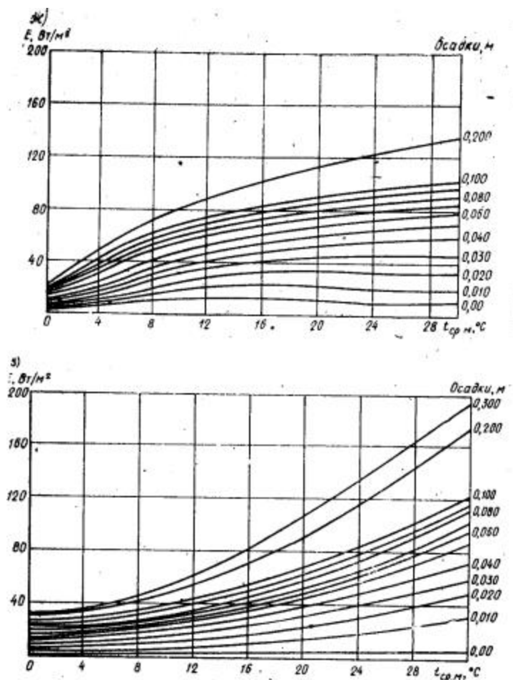
Рис. 39. Номограмма для определения затрат тепла на суммарное испарение воды с поверхности грунта по месяцам а - март; б - апрель; в - май; г - июнь; д - июль; е - август; ж - сентябрь; з - октябрь
