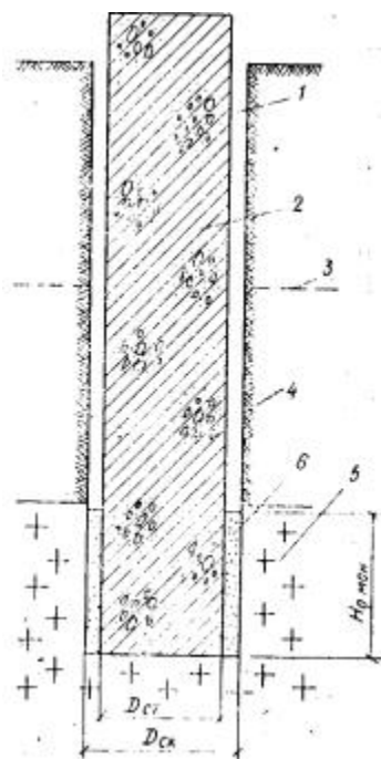
Рис. 11. Свайно-столбчатый фундамент
