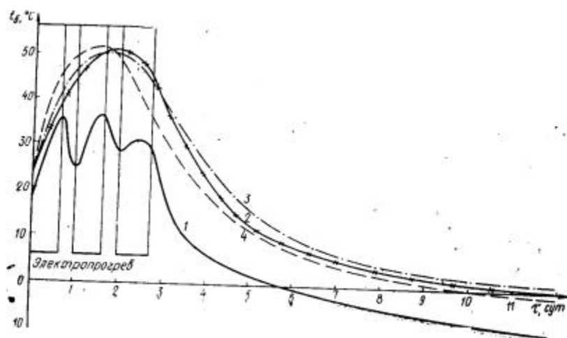
Рис. 48. Режим выдерживания бетона сваи диаметром 1000 мм
