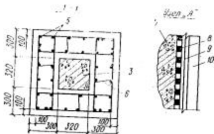
Рис. 19. Усиление свай железобетонной обоймой
