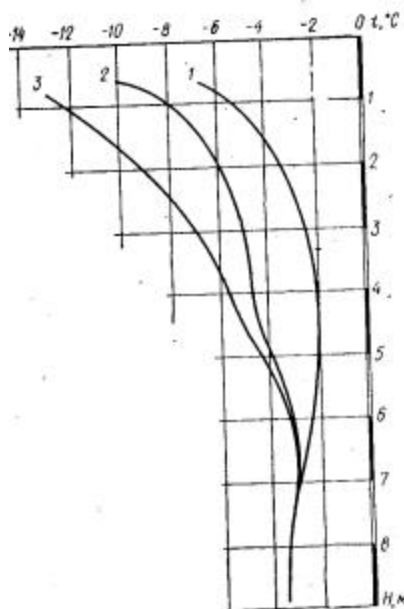
Рис. 45. График для определения температуры грунта в первой декаде февраля 1 - в естественном состоянии (со снежным покровом); 2 - на отсыпанной гравием строительной площадке (без снежного покрова); 3 - средняя по контакту с укладываемым бетоном
