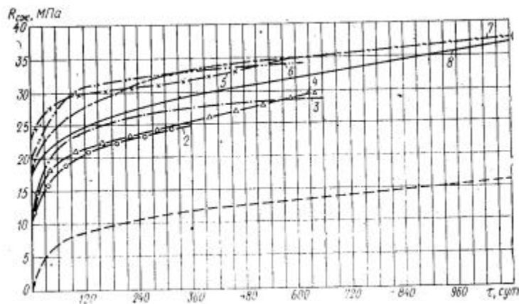
Рис. 32. Нарастание прочности бетона марки М 300 в контакте с вечномерзлым грунтом, приготовленного на портландцементе М 400-М 500 с противоморозными химическими добавками и без них
