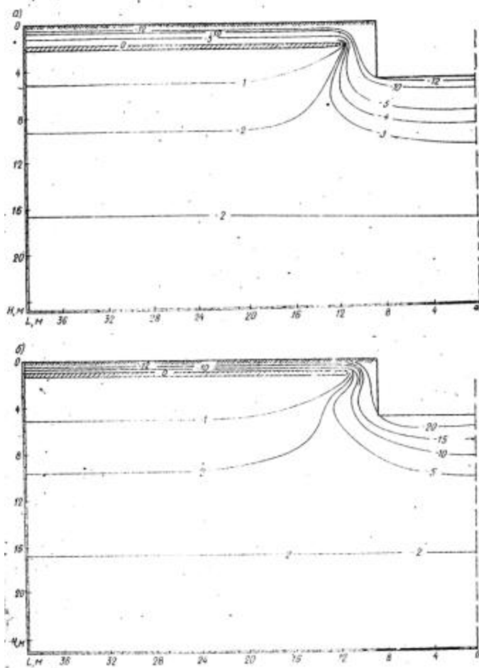
Рис. 20. Температурное поле в грунте вокруг котлована а - через 5 дней после выемки котлована; б - через 20 дней
