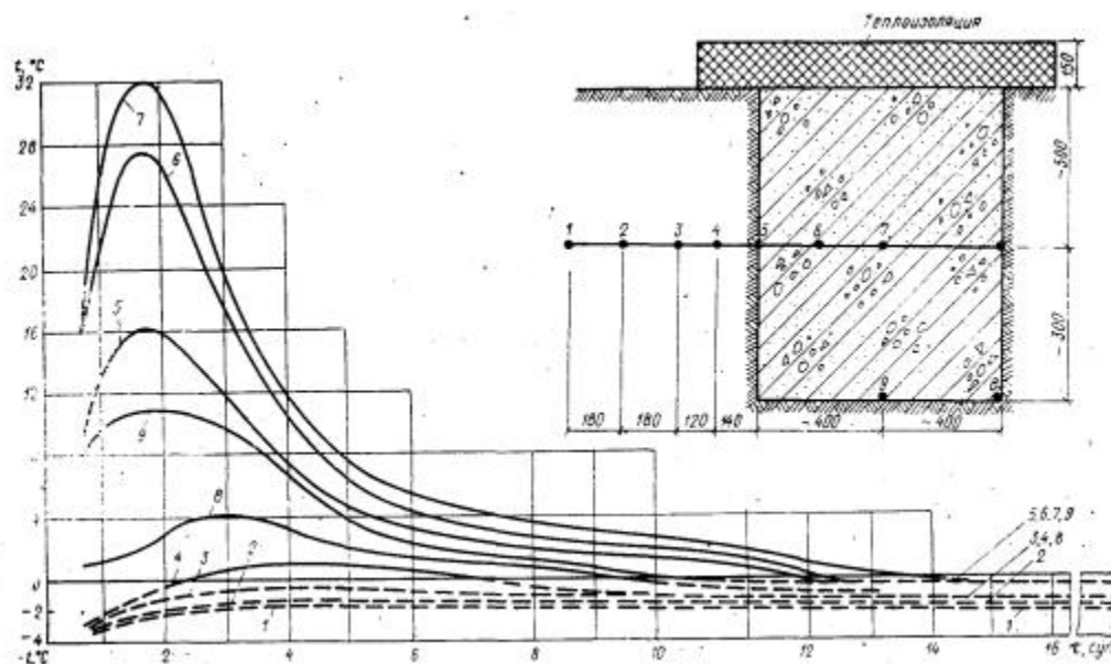
Рис. 51. Схема расположения термодпар и температурный режим остывания бетона в свае-модели диаметром 800 мм (точки и кривые 5-9) и прилегающего вечномерзлого грунта (точки и кривые 1-4)
