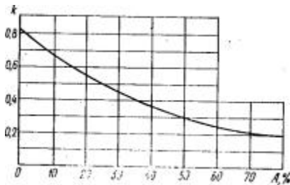
Рис. 38. График для определения коэффициента k
