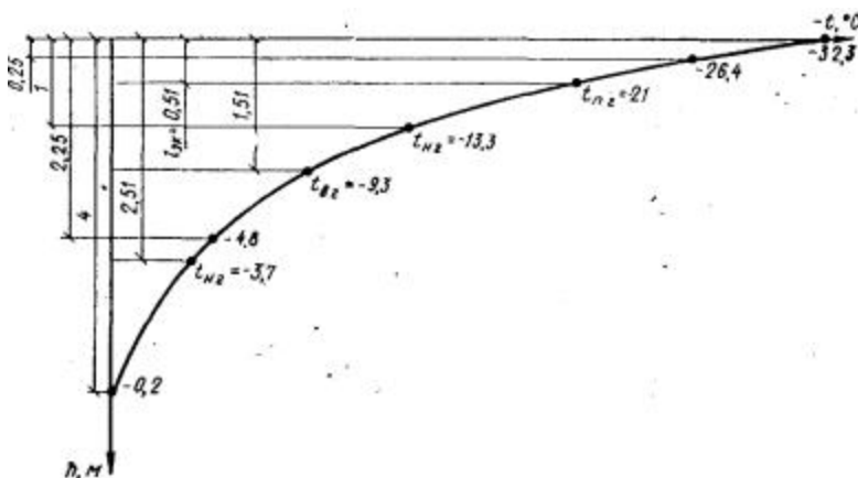
Рис. 42. График распределения температур по глубине грунта
