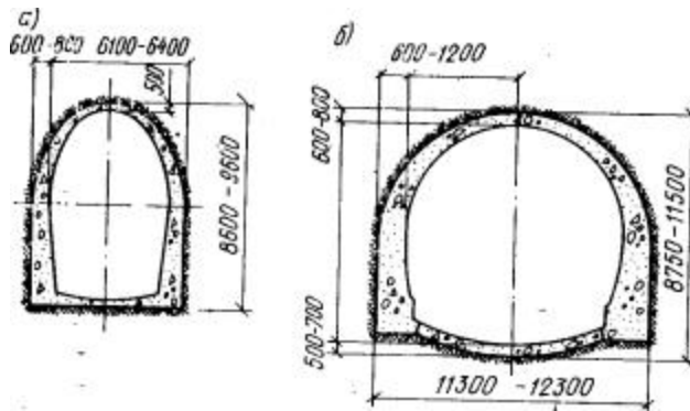
Рис. 9. Схема бетонных обделок железобетонных тоннелей а - однопутных; б - двухпутных
