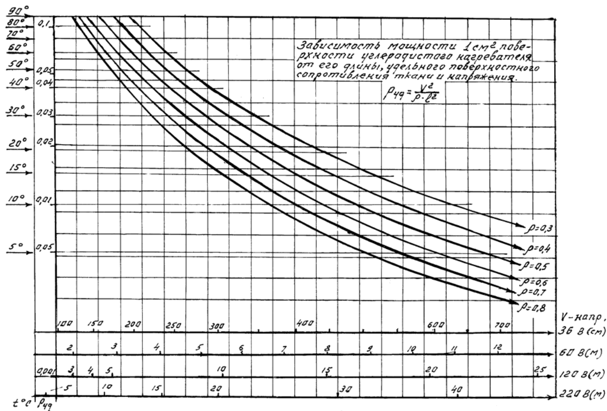
Рис. 3.3. Номограмма графического определения параметров прогрета
