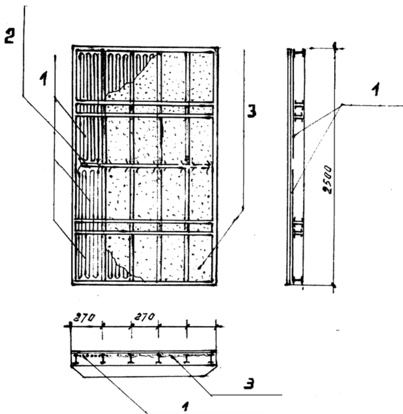
Рис. 3.6. Щит опалубки, оснащенный греющим полимерным проводом: 1 – греющий провод; 2 – подключающие провода; 3 – утеплитель (полиуретан)
