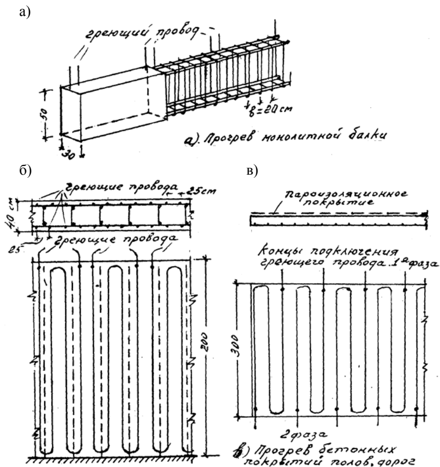
Рис. 2.7. Примеры прогрева бетона с использованием полимерного греющего провода:
