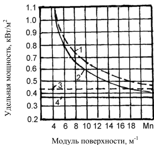
Рис. 1.4. Влияние модуля поверхности конструкции (ее массивности) на удельную мощность проволочного нагревателя при обогреве бетона, \text{кВт/м}^2 : 1 – мощность в период подъема температуры до значения экзотермического прогрева 60^\circ\text{C} ; 2 – то же до 40^\circ\text{C} ; 3 – мощность изотермического прогрева при температуре 60^\circ\text{C} ; 4 – то же при температуре 40^\circ\text{C}
