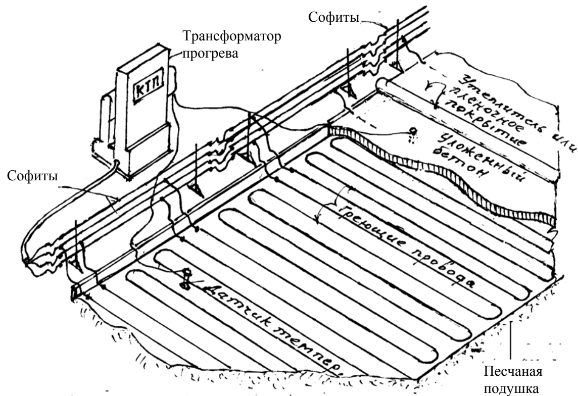
Рис. 1.6. Технологическая схема размещения проводочных нагревателей и прогрева бетона в плите
