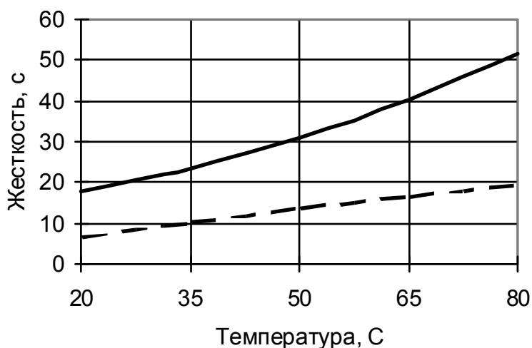
Рис. 1. Влияние температуры разогрева на жесткость сталефибробетонной смеси ( B/C = 0,55 , \mu = 1,0\% ) — без добавки; - - - с добавкой.
